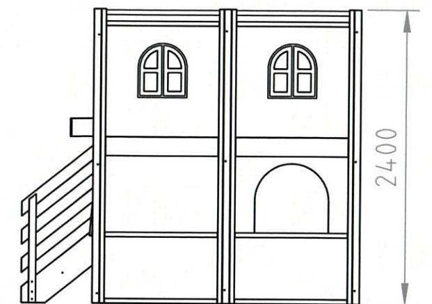
立面図 2
