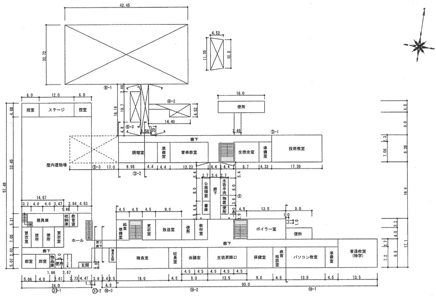
1階平面図
